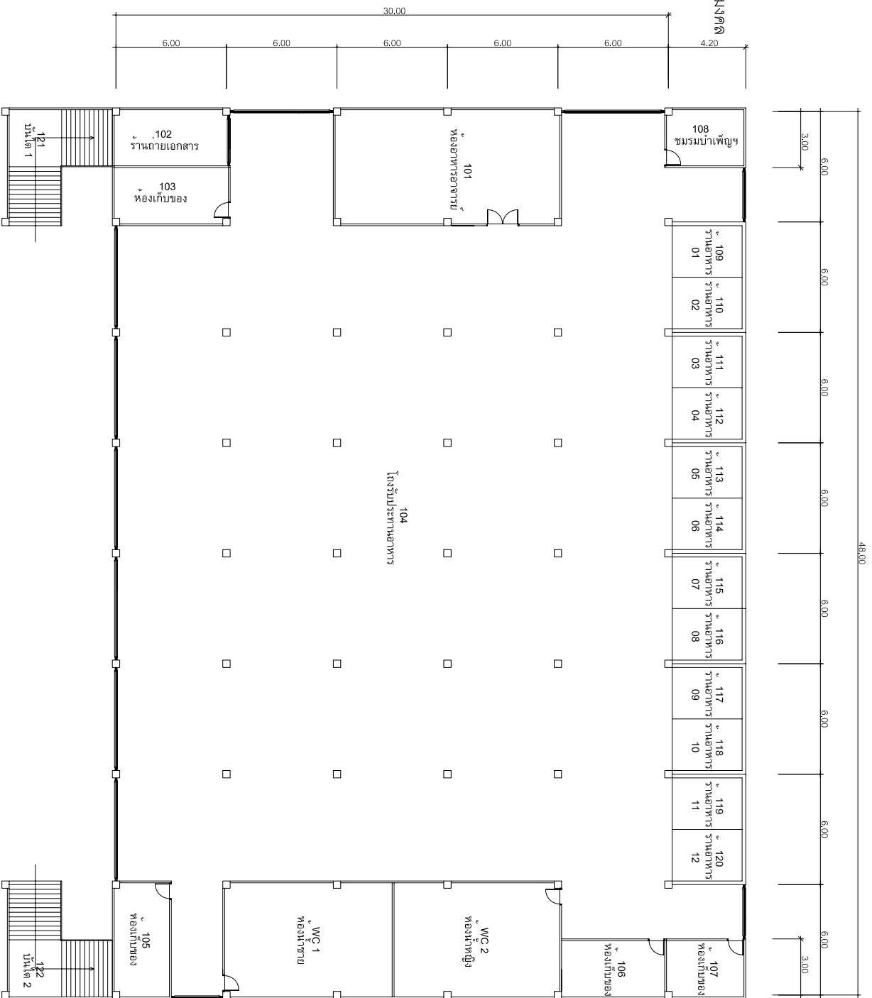
แปลนพื้นที่ชั้นกลาง อาคาร 37
