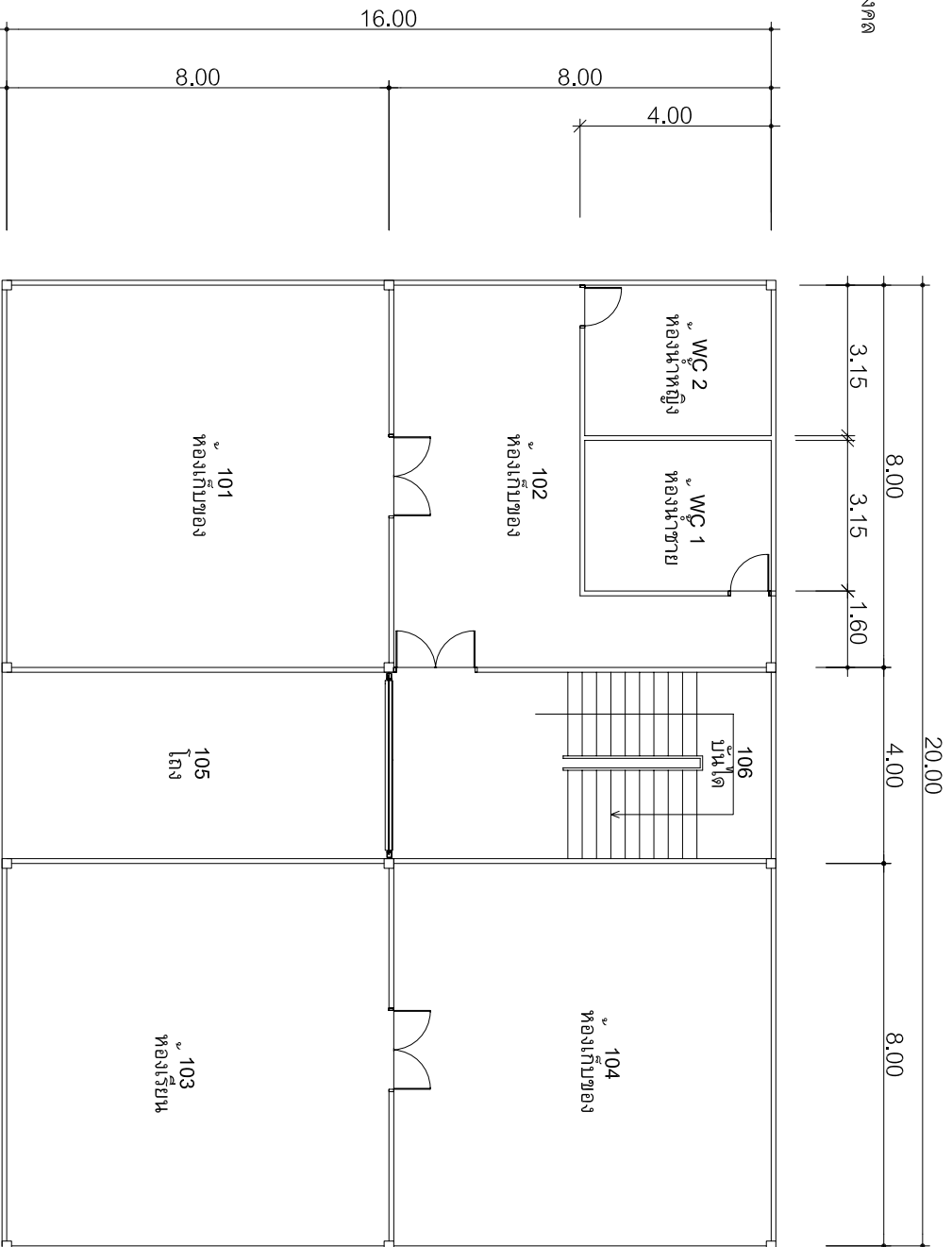
แผนชั้นล่าง อาคาร 18/4
