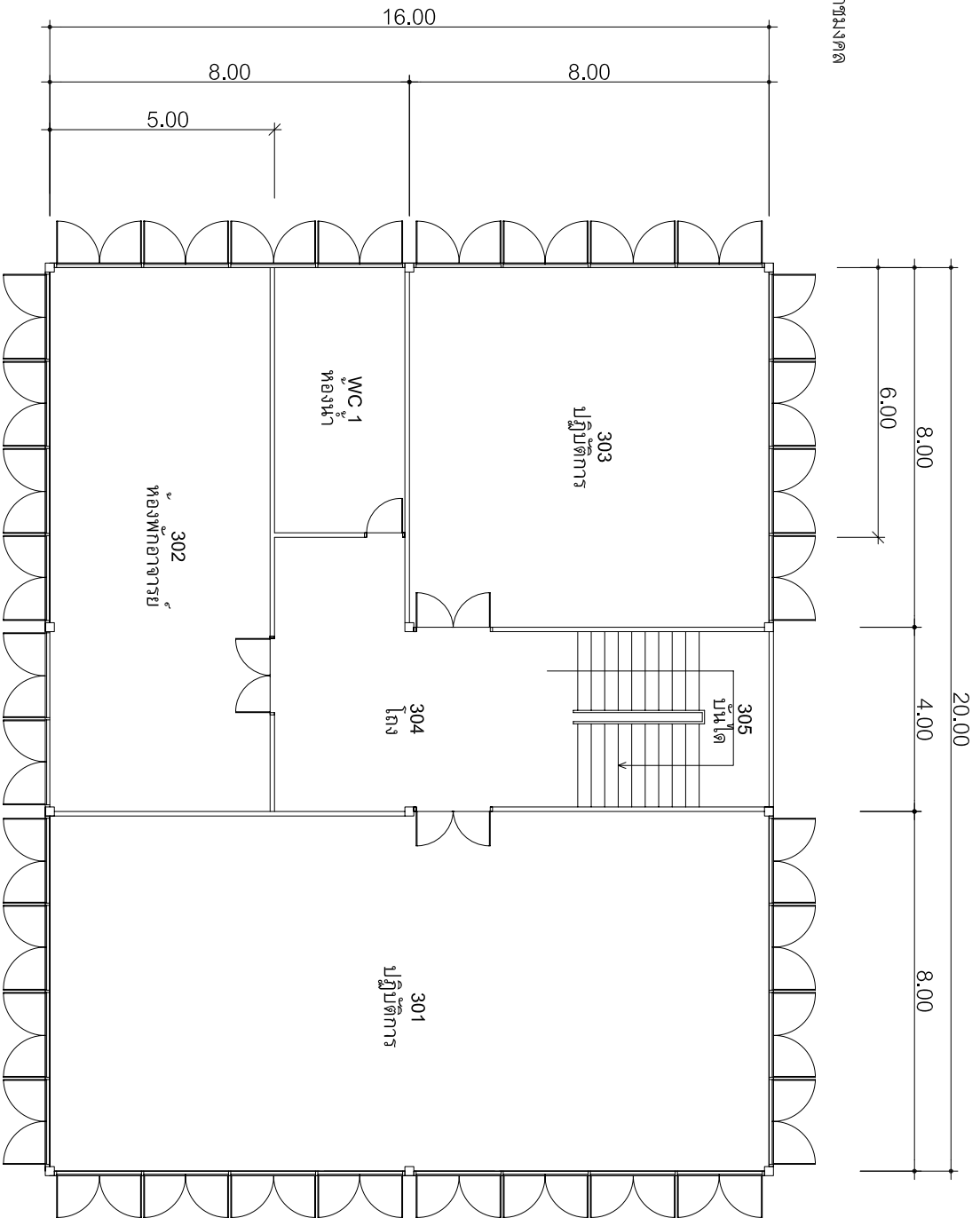
แผนชั้น 3 อาคาร 18/4
