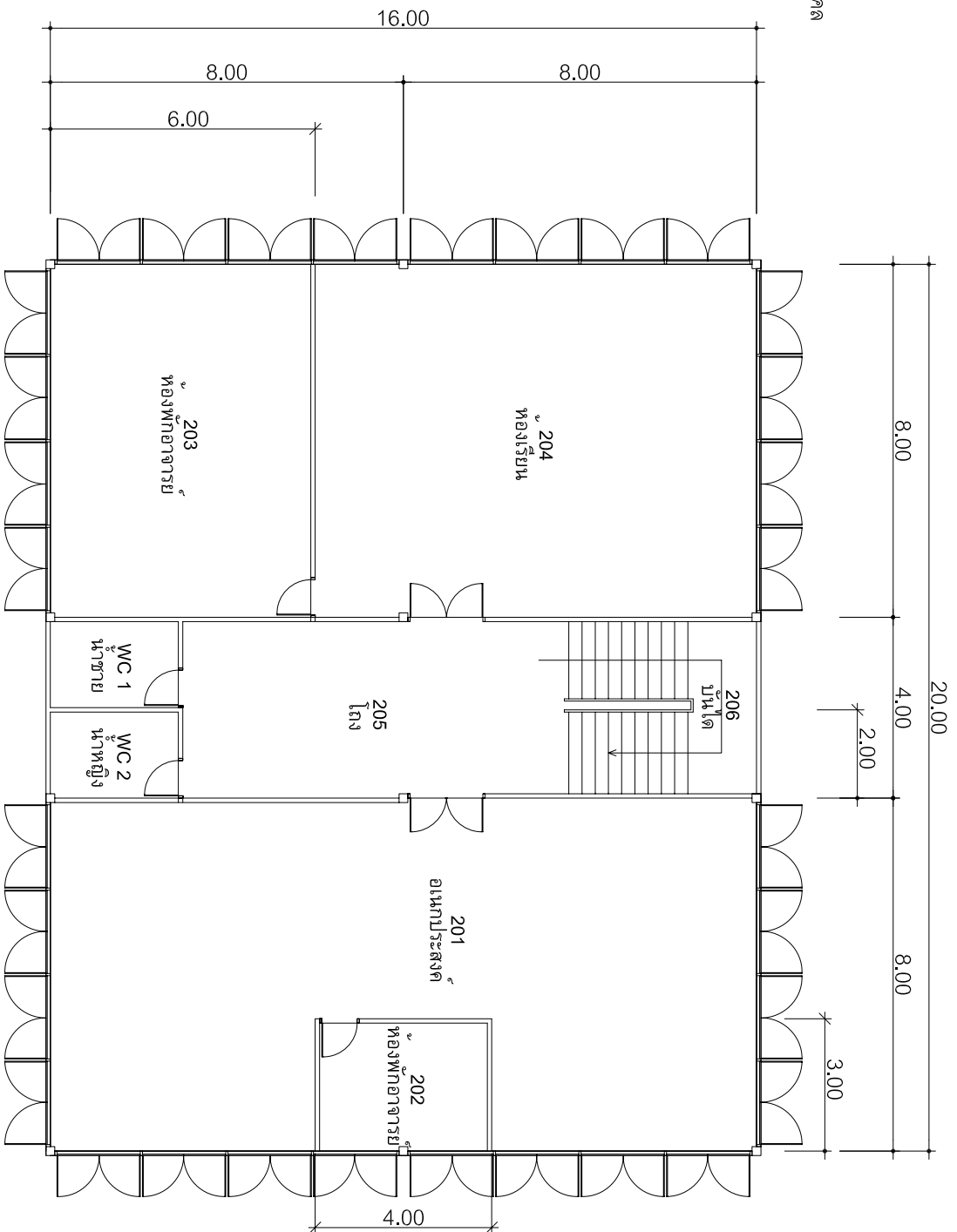
แผนชั้น 2 อาคาร 18/4
