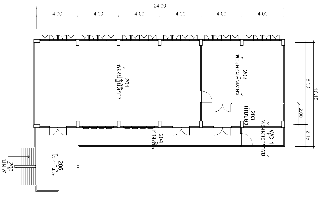
แปลนพื้นที่ชั้น 2 อาคาร 7/2
