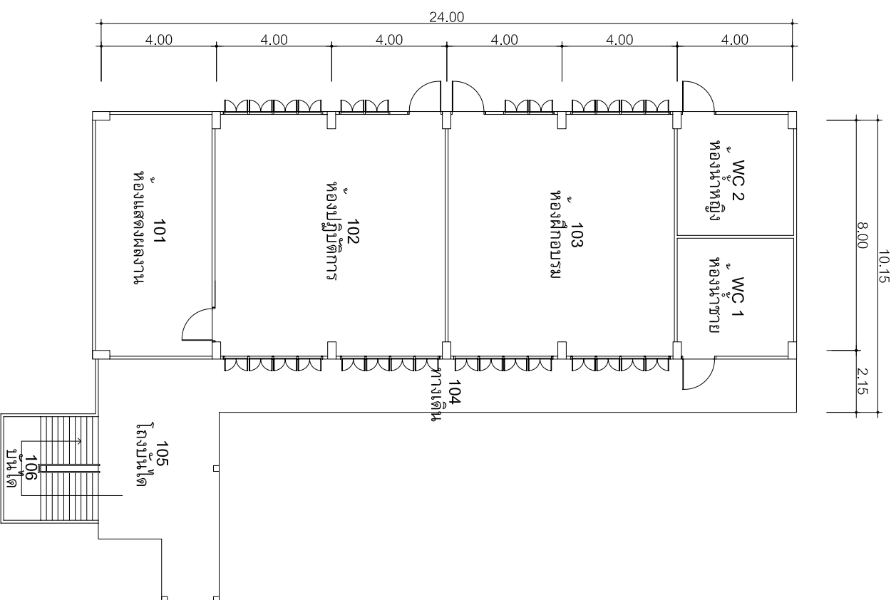
แปลนพื้นที่ชั้นล่าง อาคาร 7/2
