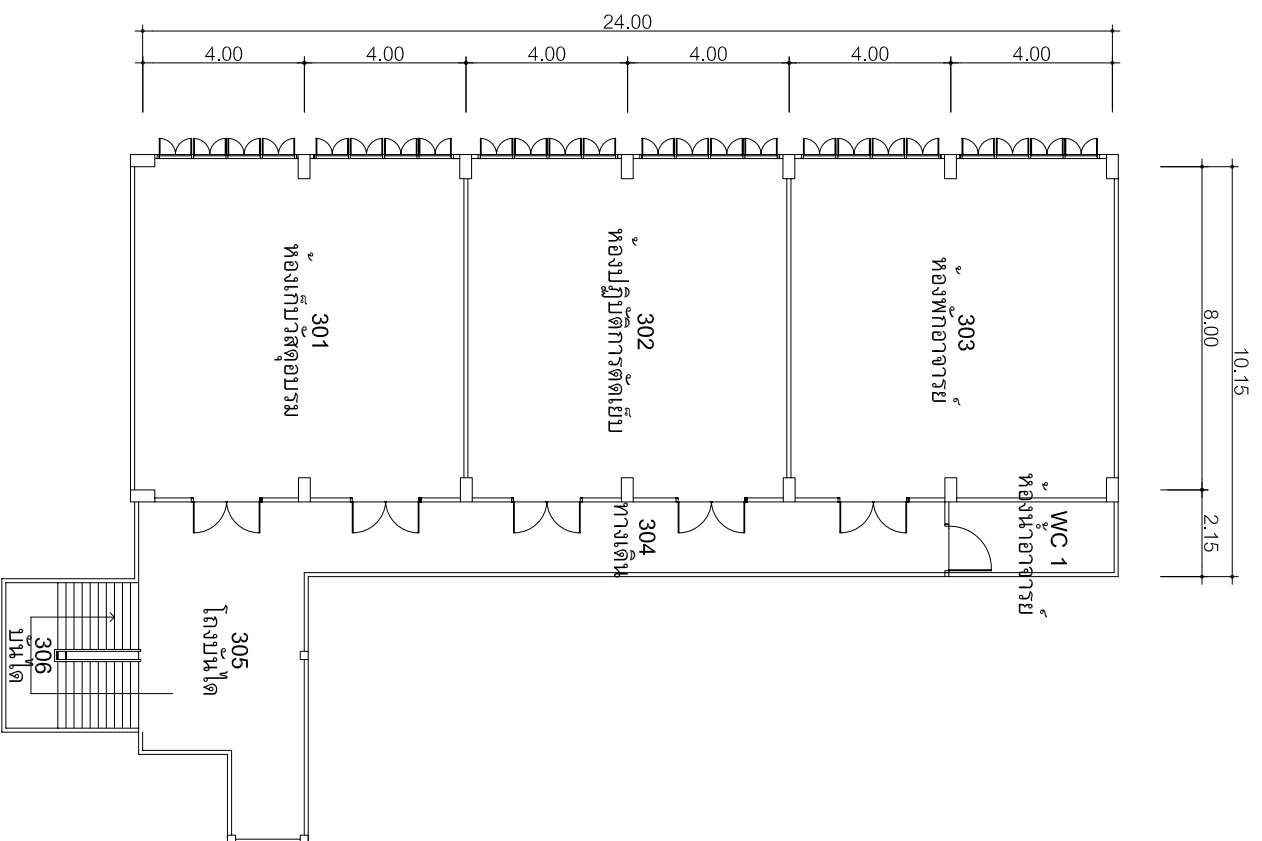
แปลนพื้นที่ชั้น 3 อาคาร 7/2
