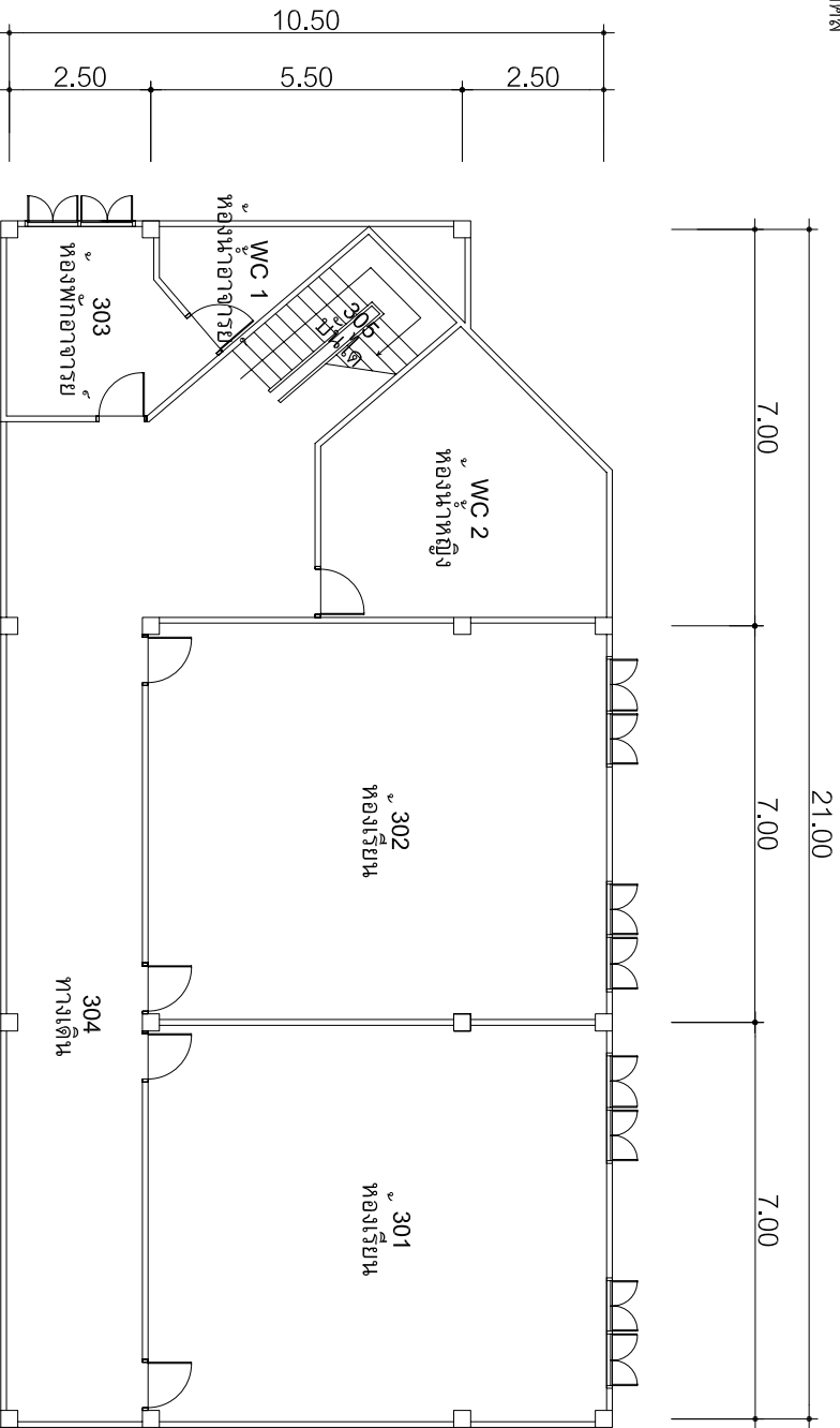
แผนผังชั้น 3 อาคาร 4/4
