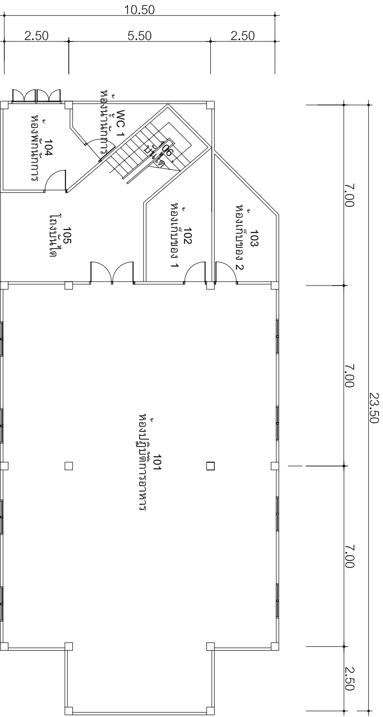
แปลนพื้นที่กลาง อาคาร 4/4
