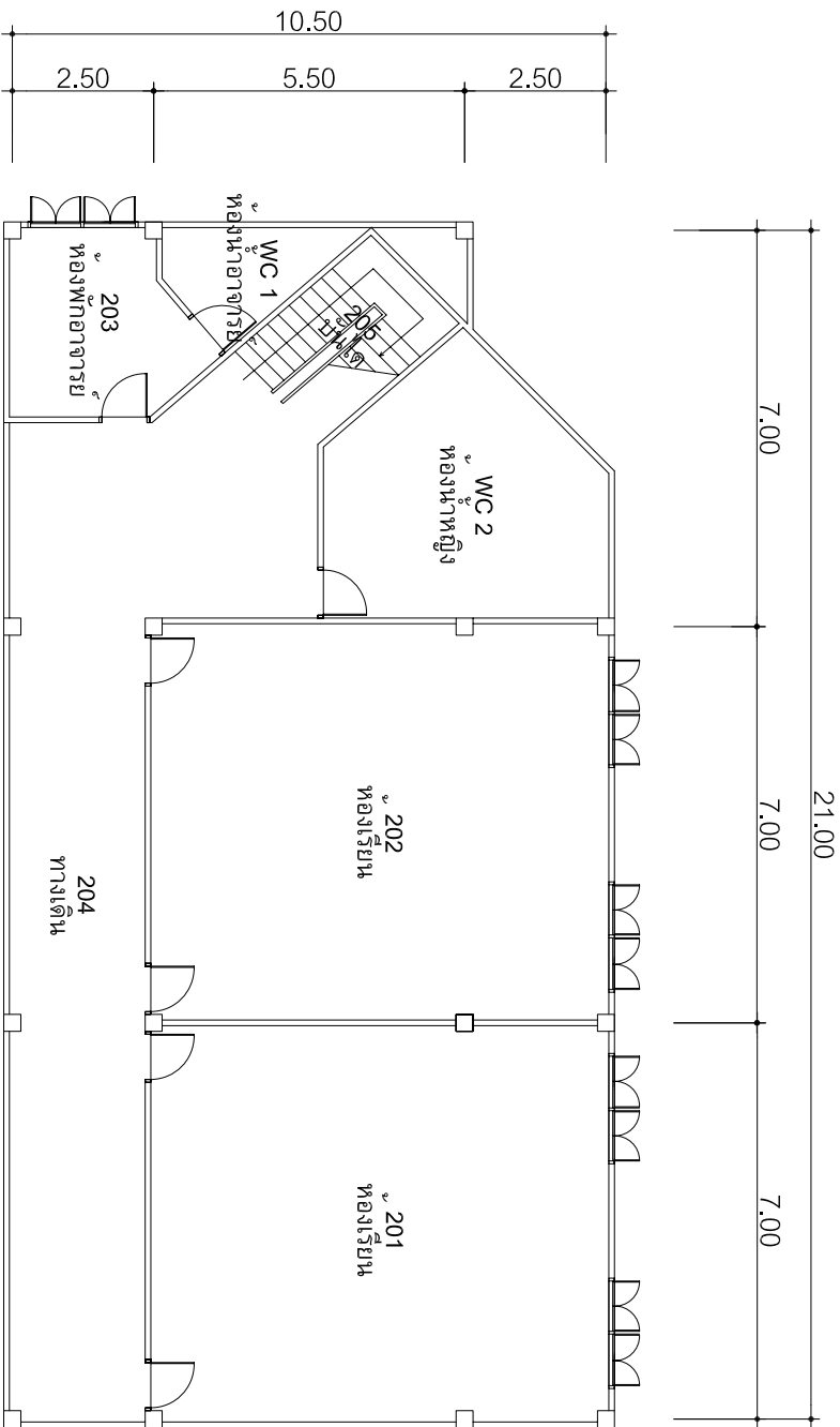
แปลนพื้นที่ 2 อาคาร 4/4
