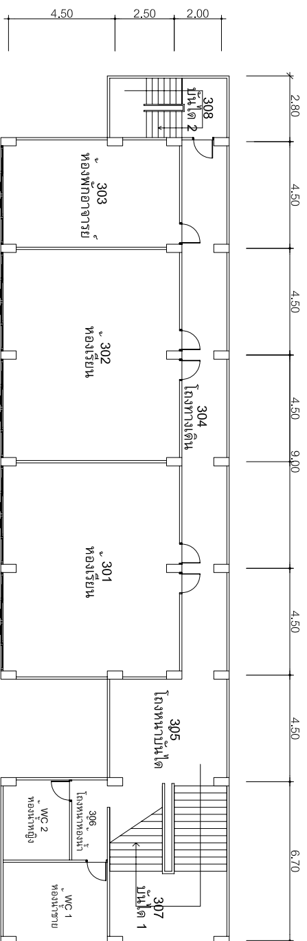
แปลนพื้นที่ 3 อาคาร 3/2
