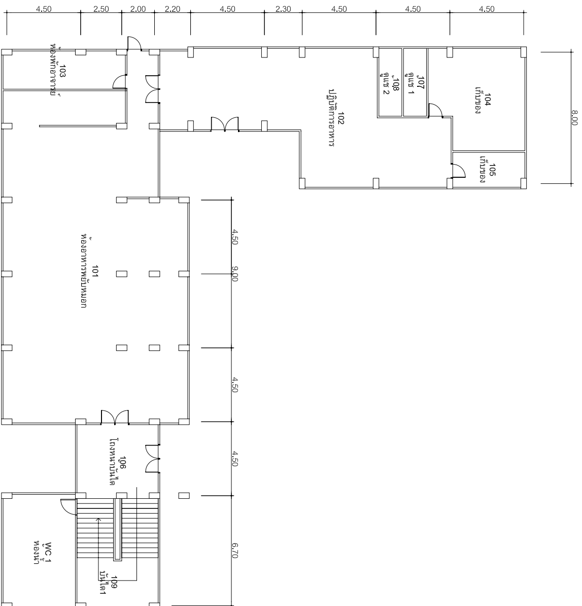
แปลนพื้นที่ชั้นล่าง อาคาร 3/2
