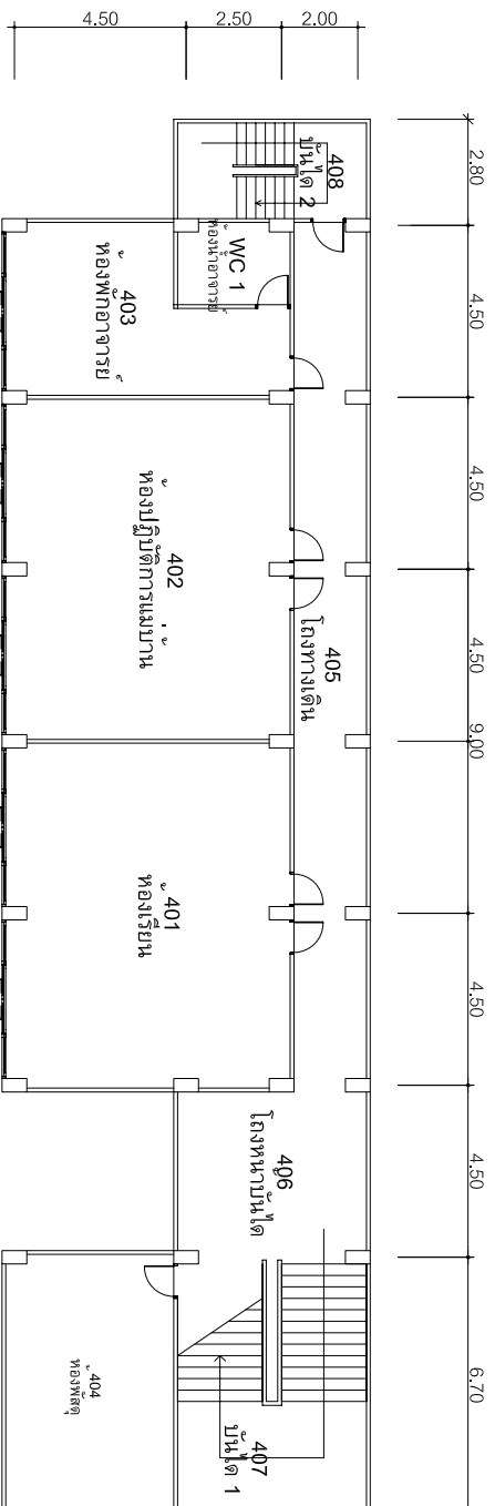
แปลนพื้นที่ 4 อาคาร 3/2
