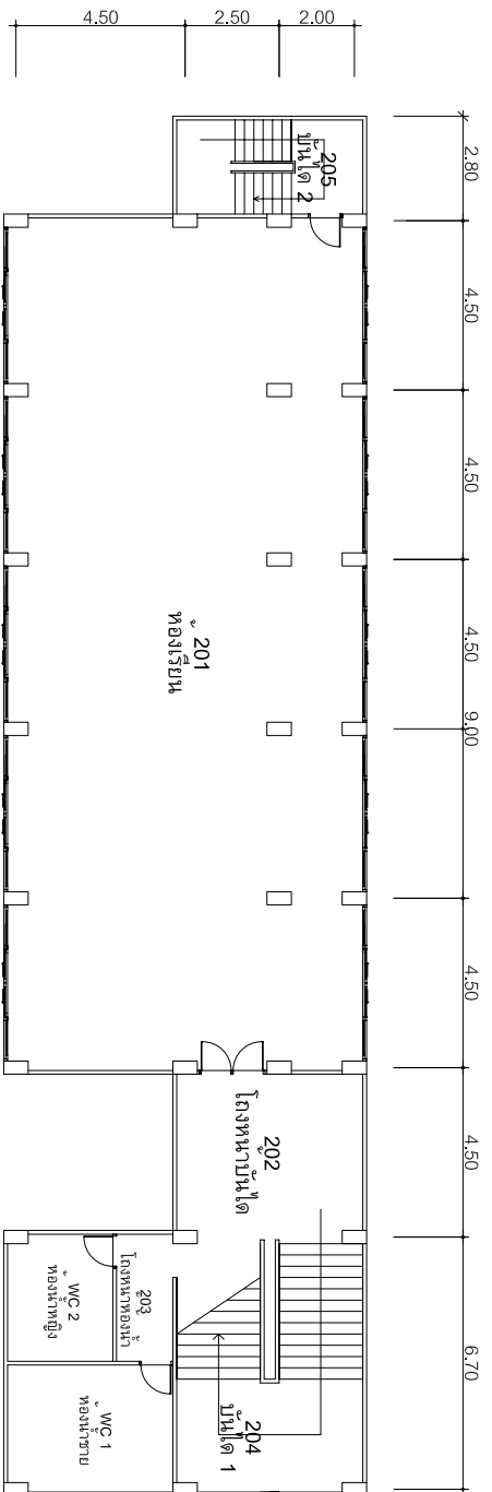
แปลนพื้นที่ชั้นที่ 2 อาคาร 3/2
