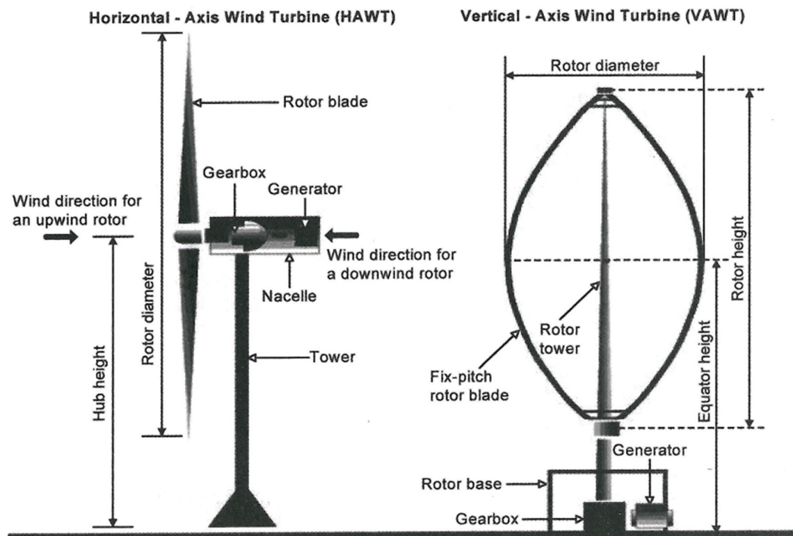
กังหันลมแกนหมุนแนวตั้ง
