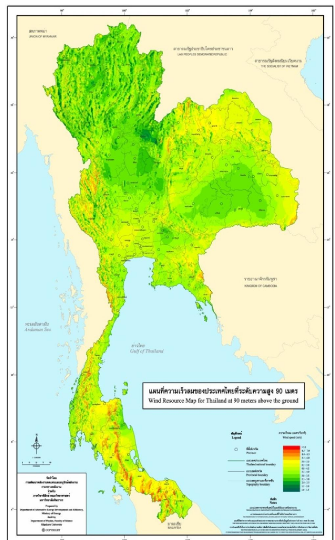
แผนที่ความเร็วลมของประเทศไทยที่ระดับความสูง 90 เมตร
