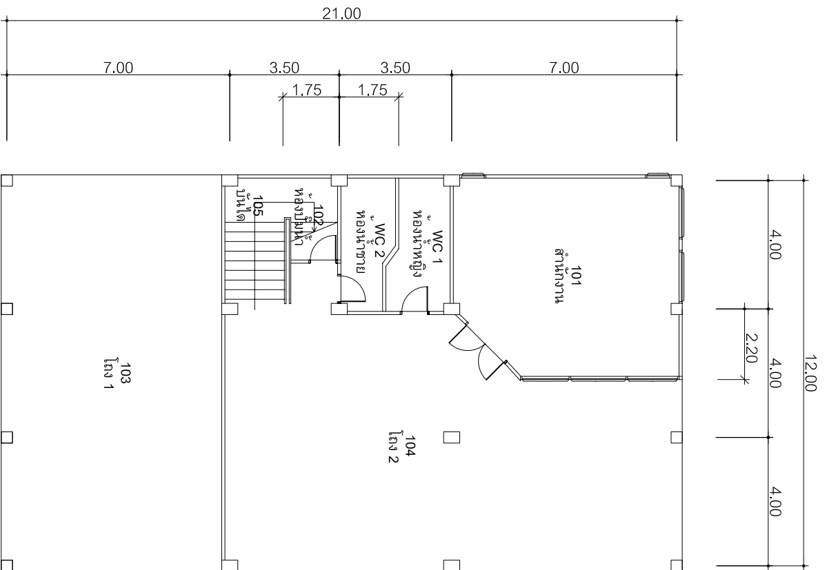
แปลนชั้นล่าง อาคาร 16/3
