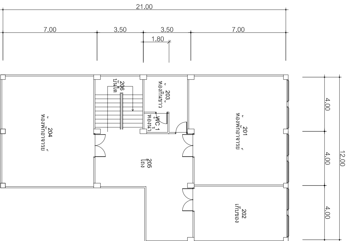
แปลนชั้น 2 อาคาร 16/3
