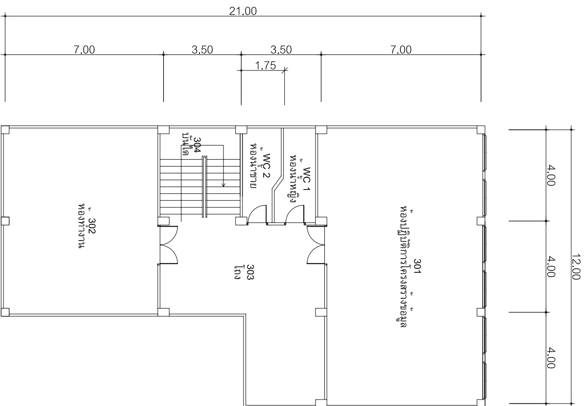
แปลนชั้น 3 อาคาร 16/3
