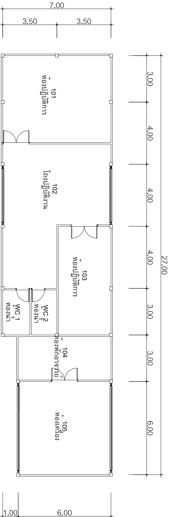
แปลนอาคาร 15/4
